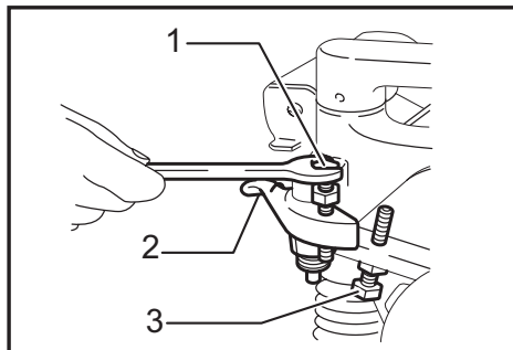
► 1. Ajuste del perno hexagonal para la posición predeterminada No. 1 2. Palanca (C) 3. Ajuste del perno hexagonal para la posición predeterminada No. 2
