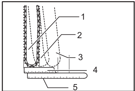
► 1. Posición original 2. Posición predeterminada No. 1 3. Posición predeterminada No. 2 4. Placa de indicación 5. Regla
